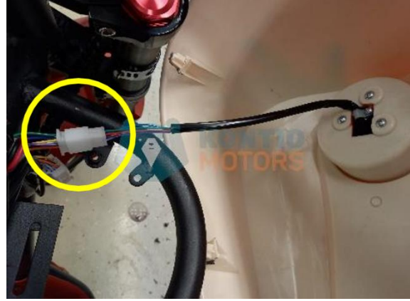
Irrota yläkannessa oleva mittarin johto.
