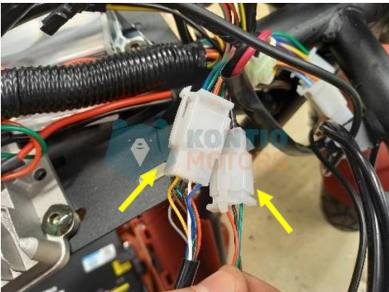
Seuraa kaasukahvan johtoja kahvalta tankille. Irrota kaasukahvalta tulevien kahden johdon liittimet.
